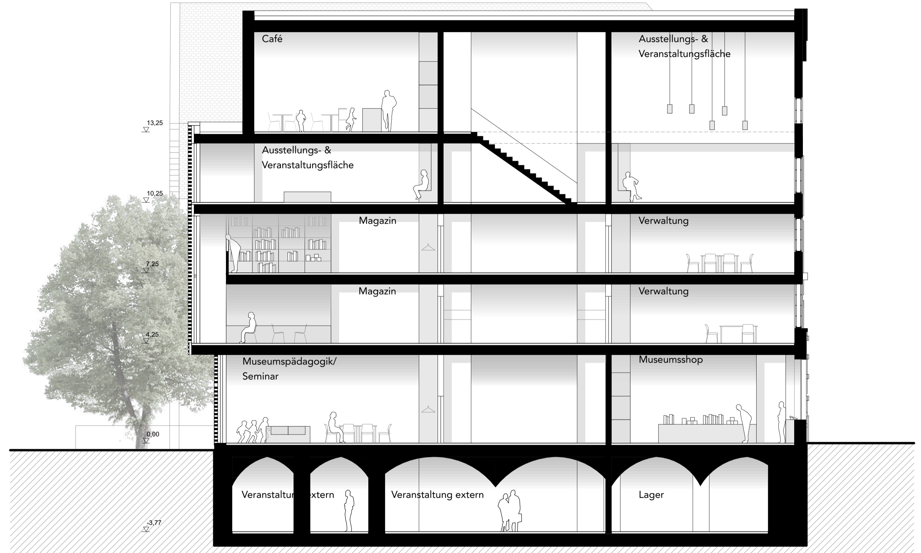
Längsschnitt BB M 1:100
